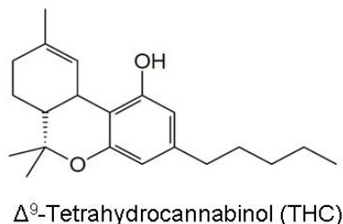
Figuur I-3 Structuurformule van \Delta^9 -tetrahydrocannabinol (THC).
