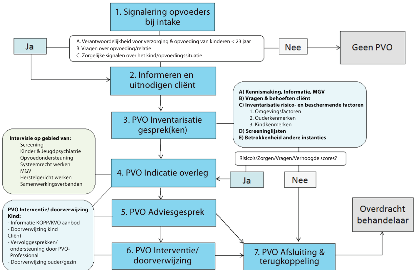
Figuur 1. Stappenschema
